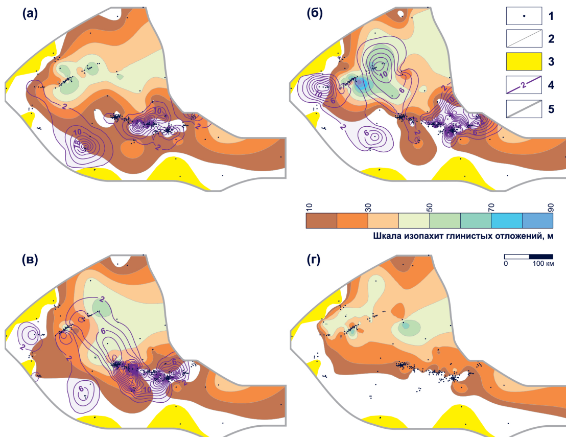
Рис. 7. Карты изопахит глинистых пород мономской свиты, перекрывающих песчаные пласты (а) T_1-I , (б) T_1-Ia , (в) T_1-II мономской свиты и (г) T_1-III таганджинской свиты: 1 – скважина; 2 – изопахиты глинистых отложений, м; 3 – зона отсутствия мономской свиты; 4 – изопахиты песчаных пластов-линз, м; 5 – полигон исследования
