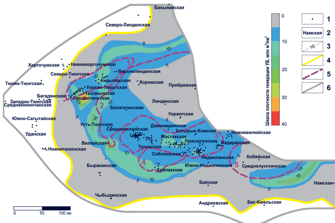
Рис. 5. Карта суммарных масштабов генерации УВ органическим веществом в нижней и средней частях газопродуцирующих отложений перми от момента литификации флюидоупоров нижнего триаса до настоящего времени (205–0 млн л): 1 – скважина; 2 – название площади бурения; 3 – изолинии плотности генерации УВ, млн м 3 /км 2 ; границы: 4 – отсутствия газопродуцирующих отложений перми, 5 – структур I-II порядка по отражающему горизонту ТП (1 – Логлорский вал, 2 – Линденская впадина, 3 – Хапчагайский мегавал, 4 – Тангарынская впадина, 5 – Лунгхинско-Келинская впадина); 6 – полигон исследования
