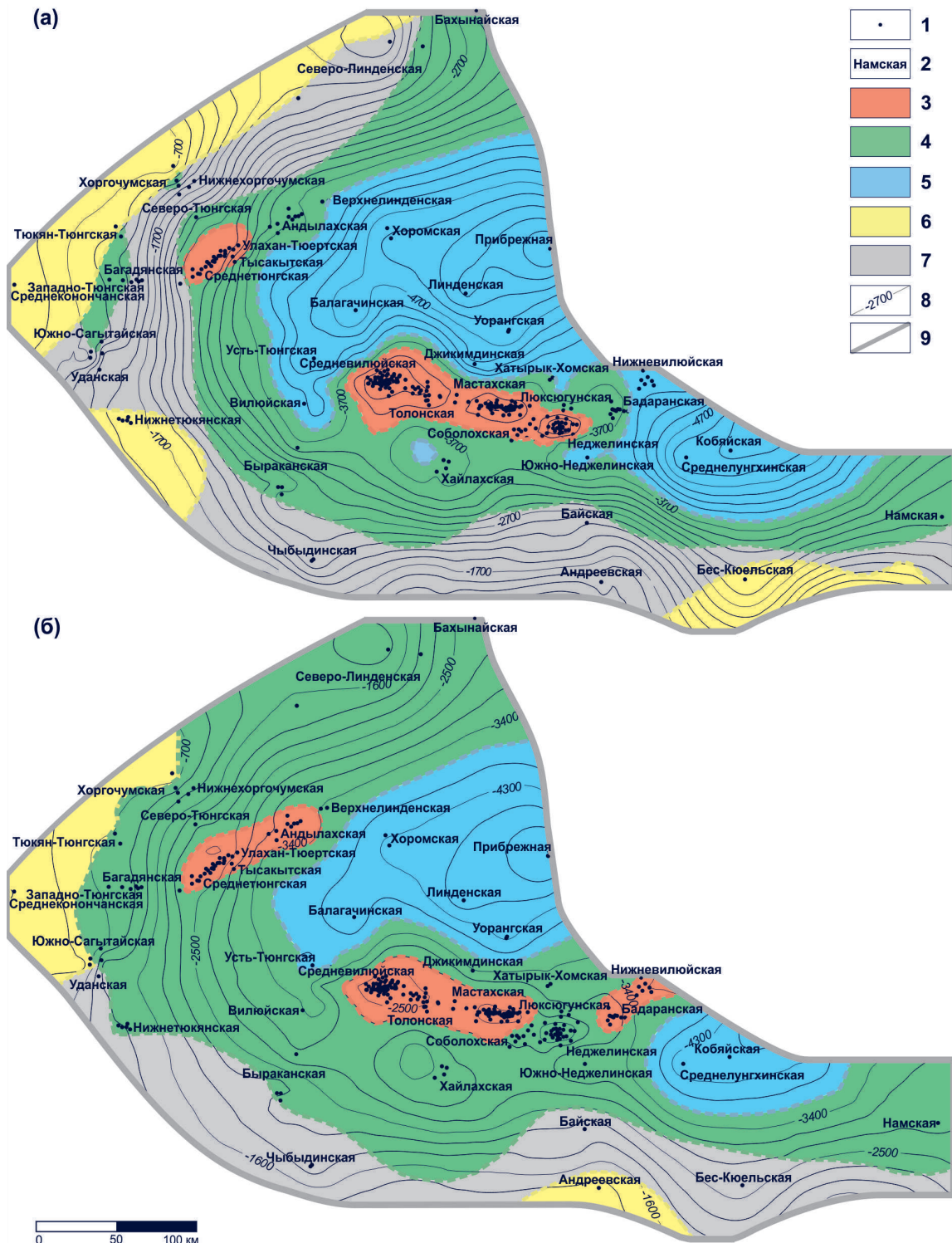
Рис. 9. Карты перспектив нефтегазоносности (а) верхнепермско-нижнетриасового и (б) нижнетриасового нефтегазоносных комплексов: 1 – скважина; 2 – название площади бурения; земли: 3 – перспективные с доказанной промышленной газоносностью, 4 – перспективные, 5 – низкоперспективные, 6 – бесперспективные, 7 – невыясненных перспектив; 8 – изогипсы, м (кровля (а) верхнепермских, (б) нижнетриасовых отложений); 9 – полигон исследования.
