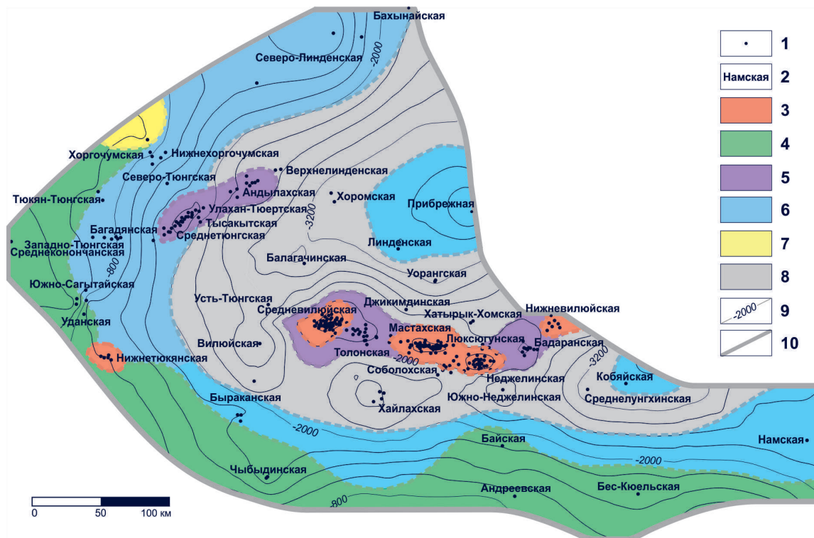
Рис. 10. Карта перспектив нефтегазоносности нижнеюрского нефтегазоносного комплекса: 1 – скважина; 2 – название площади бурения; земли: 3 – перспективные с доказанной промышленной газоносностью, 4 – перспективные, 5 – потенциально перспективные, 6 – низкоперспективные, 7 – бесперспективные, 8 – невыясненных перспектив; 9 – изогипсы, м (кровля нижнеюрских отложений); 10 – полигон исследования.
