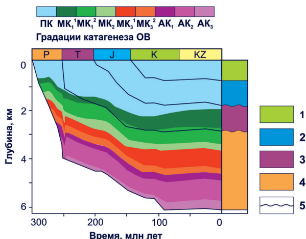
Рис. 4. История погружения осадочных комплексов и изменения катагенетической преобразованности ОВ в разрезе Хапчагайского мегавала: 1 – меловые, 2 – юрские, 3 – триасовые, 4 – газоматеринские пермские отложения; 5 – несогласное залегание пород
