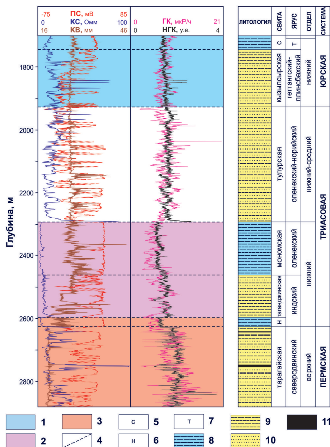
Рис. 2. Опорный разрез верхнепалеозойских и мезозойских отложений (скв. Северо-Тюнгская № 222): 1 – нижнеюрский, 2 – нижнетриасовый, 3 – верхнепермско-нижнетриасовый нефтегазоносные комплексы; 4 – границы литостратиграфических подразделений; 5 – сунтарская, 6 – неджелинская свиты; 7 – тоарский ярус; 8 – аргиллиты; 9 – алевролиты; 10 – песчаники; 11 – угли
