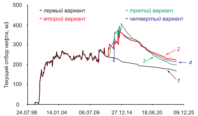
Рис. 8. Текущий отбор нефти по вариантам разработки.
